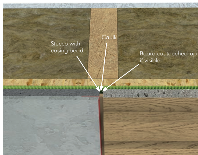
Fig. 29 - Abutting stucco
