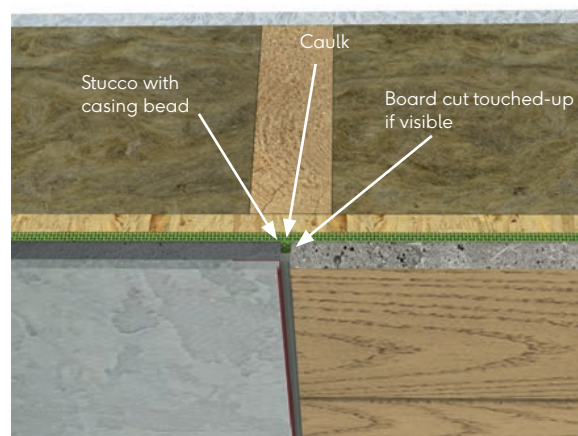
Fig.31 - Abutting stucco
